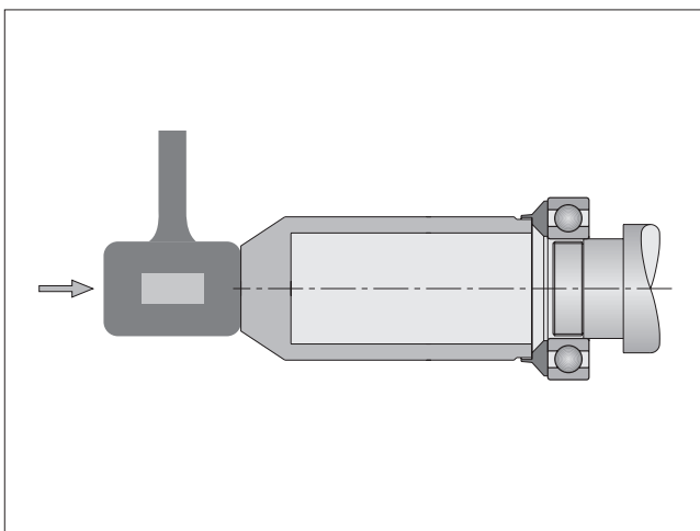
Mit geeigneten Schlagbüchsen, wie sie in den FAG Einbauwerkzeugsätzen enthalten sind, treibt man kleine Lager mit leichten Hammerschlägen auf.
